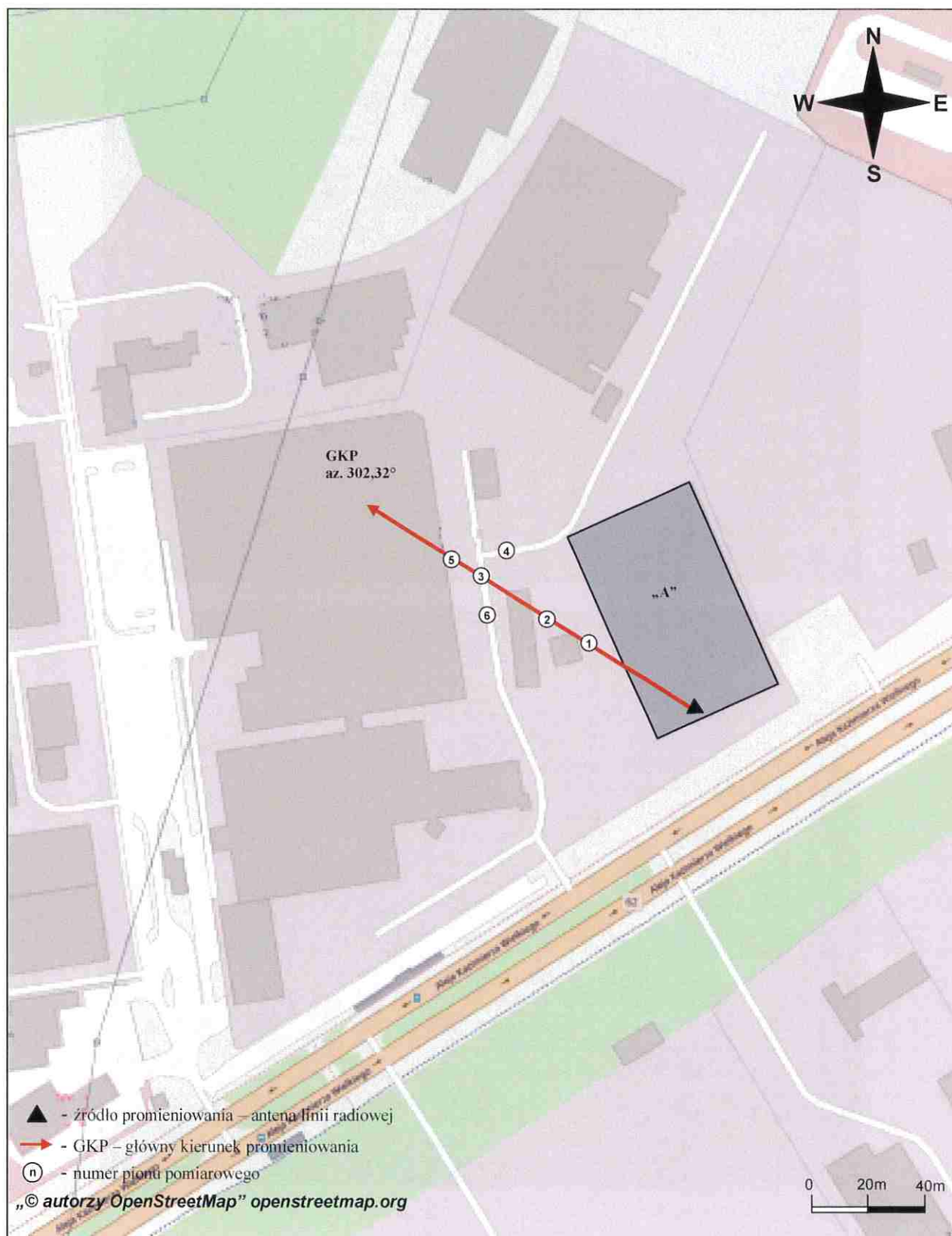
Rys. 1. Usytuowanie punktów i pionów pomiarowych w otoczeniu instalacji radiokomunikacyjnej Stacja Netia WLOEB252-WLOEM00028 Włocławek, Aleja Kazimierza Wielkiego 6
