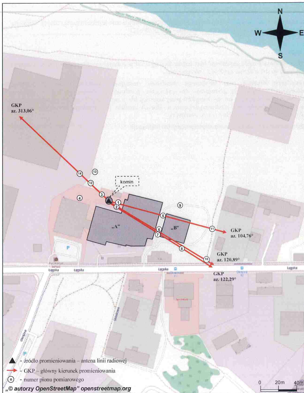
Rys. 1. Usytuowanie punktów i pionów pomiarowych w otoczeniu instalacji radiokomunikacyjnej Stacja Netia WLOEB092-WLOEM00015 Włocławek, ul. Lęska 16
